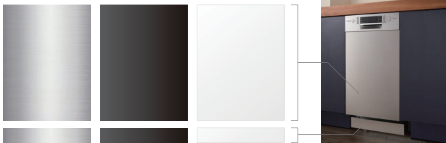
面材 ステンレス【HL仕上】: 幅444(446)mm×高さ590mm×厚さ19mm ※( )は戸当たりゴムを含めた寸法 マットブラック/マットホワイト: 幅444mm×高さ590mm×厚さ19.6mm 巾木 ステンレス【HL仕上】/マットブラック/マットホワイト 幅446mm×高さ75mm×厚さ18.3mm ステンレス面材+巾木セット: 30,000円(税別) マットブラック面材+巾木セット: 20,000円(税別) マットホワイト面材+巾木セット: 20,000円(税別)
