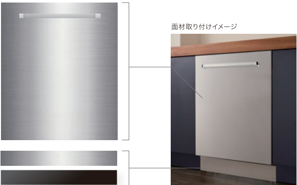
面材(ステンレスハンドル付) ステンレス【HL仕上】: 幅594(596)mm×高さ704mm×厚さ19mm ハンドル: 幅412mm×高さ22mm×奥行き37mm ハンドル厚さ12mm ※( )は戸当たりゴムを含めた寸法 巾木 ステンレス【HL仕上】: 幅596mm×高さ75mm×厚さ18.3mm 黒ポリ【アイカポリ黒ツヤ消し】: 幅596mm×高さ75mm×厚さ17mm 面材+ステンレス巾木セット: 42,000円(税別) 面材+黒ポリ巾木セット: 39,000円(税別)
